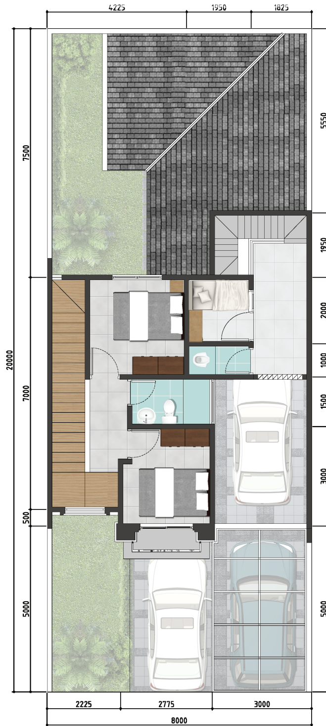
DENAH LANTAI ATAS SKALA 1:100
